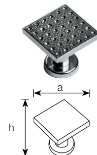
Ручка-кнопка BY21238
