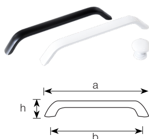
Ручка BY28003
