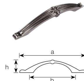
Ручка BY28095
