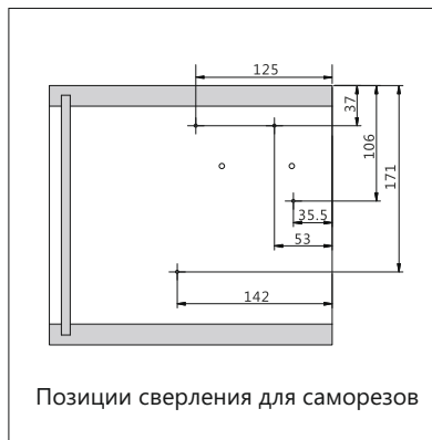
Позиции сверления для штифтов
